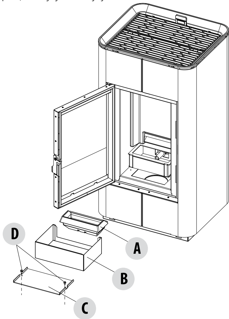
REINIGUNG DES UNTEREN FACHS - SIEHE ABBILDUNG OFEN TRAY
