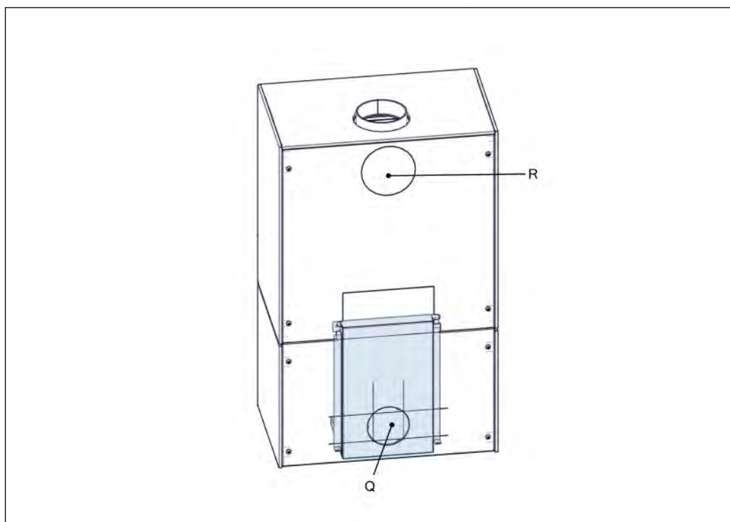
Abbildung 6. Rückansicht der BOX 20 67 mit Holzscheit-Speichermodule
